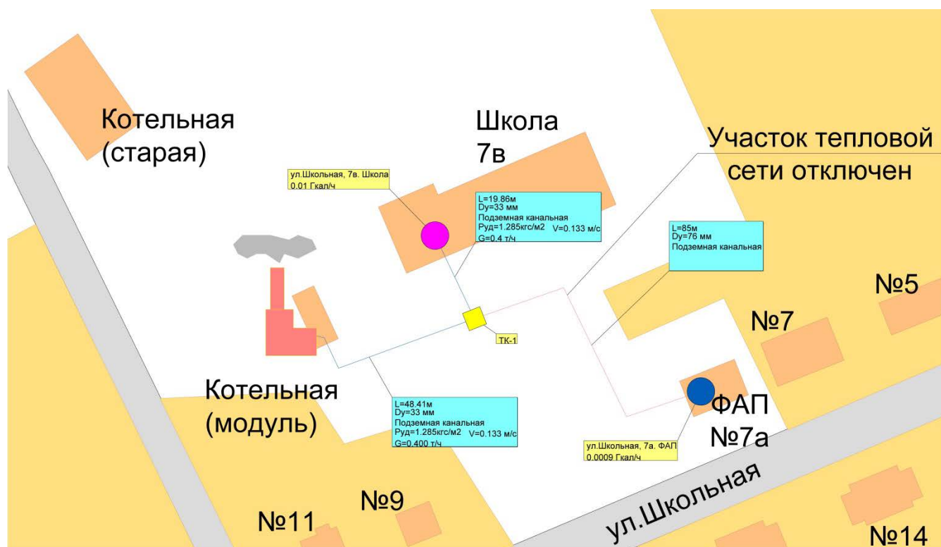
Рисунок 2.2 – Зона действия и схема тепловых сетей котельной п. Тополевка с учетом перспективы
