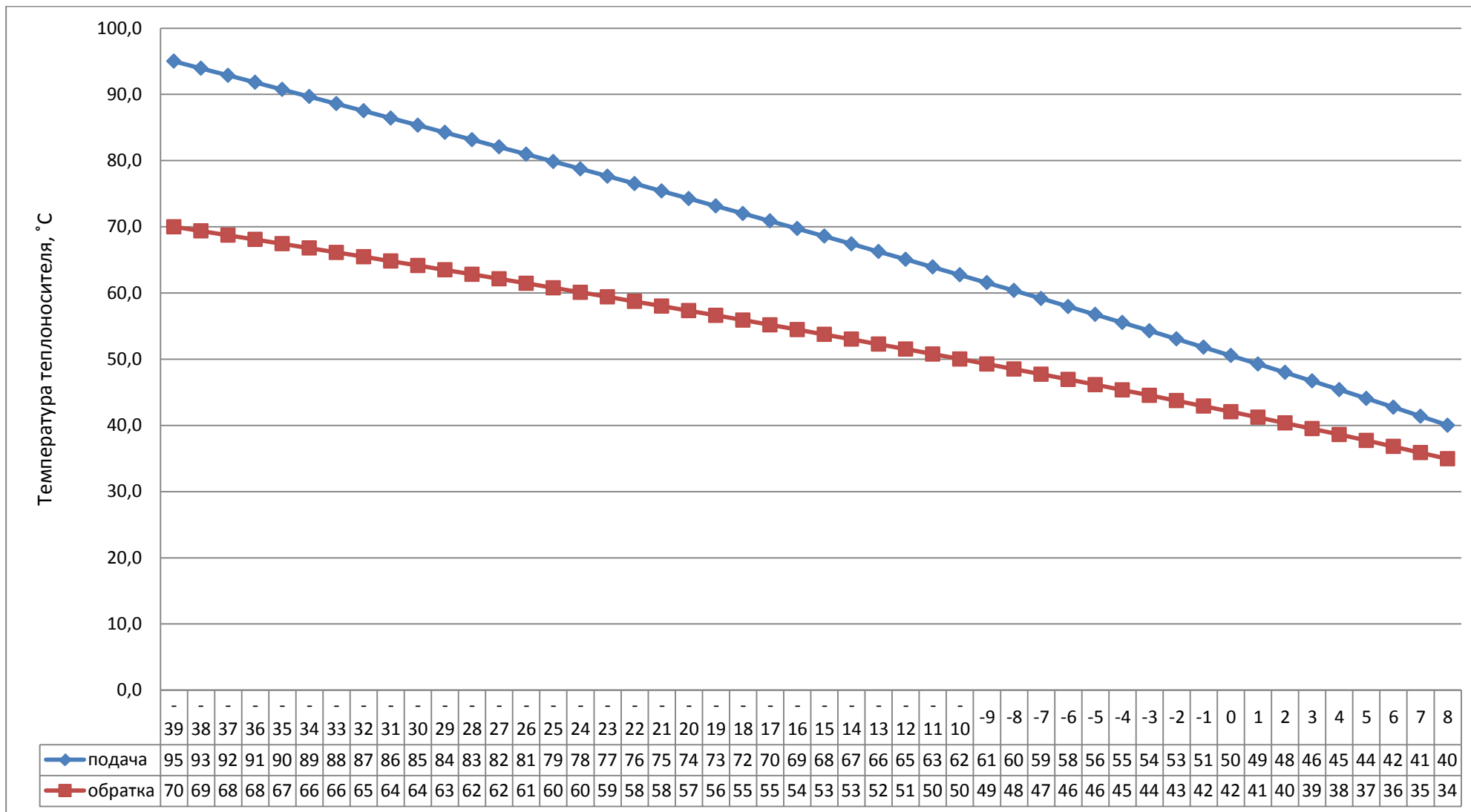
Рисунок 4.1 – Температурный график 95/70 °С
